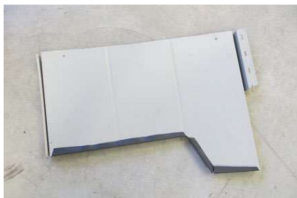
Obr. b – Úprava třetí šablony krytiny Classic ze spodní strany.
