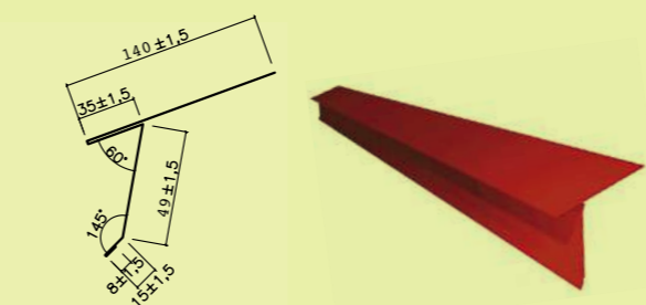
Okapové lemování prodloužené RA1AECZ krycí délka 1900 mm
