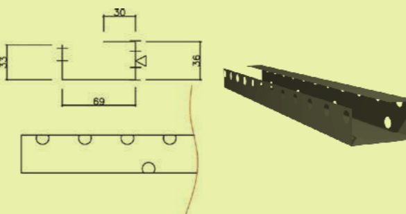
Větrací lišta RA1AS460 délka 460 mm pro hřebenáč vodorovný a 3000 mm pro hřebenáč šikmý (nároží)
