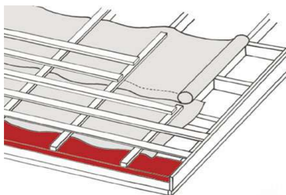
Příklad pokládky fólie
