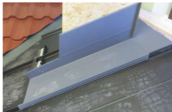
Obr. d – Na připravenou první šablonu krytiny Classic osadíme druhou, která bude tvořit boční část oplechování komínu. V místě přeložení druhé a třetí šablony jsou vnější strany zámků opět odstříhnuté.
