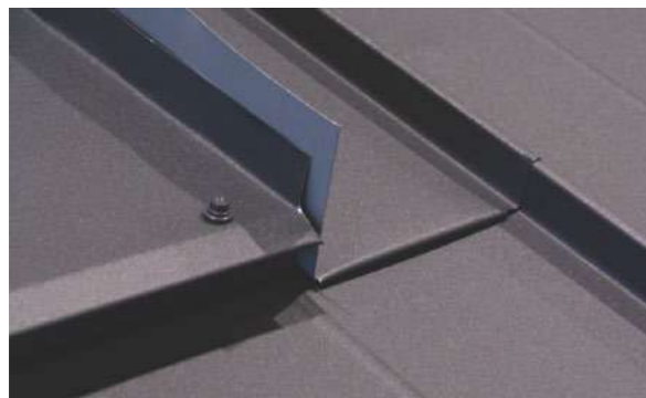
Klempířské spojení čelního oplechování a boční šablony.
