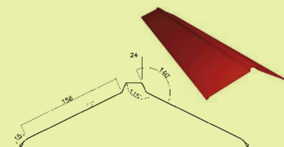
Hřebenáč hladký RA9AR krycí délka 1900 mm
